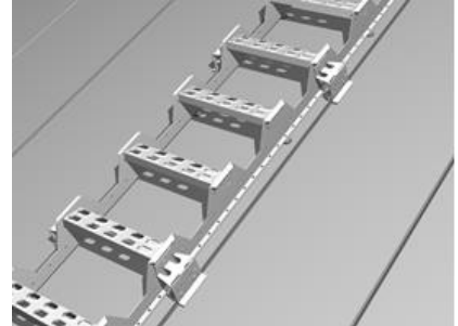
Kuva 3. Kone- ja lukkosauma-katto
