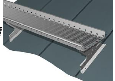
Kuva 3. Kone- tai lukkosauma
