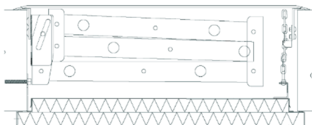
5. Tuletõkkega rõduluugi läbilõige
