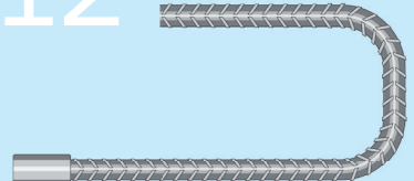
U-Muffenstab
