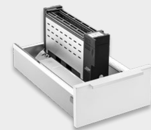
Schubladenausbau Toaster Stahl Silber 230V ab Breite 300 mm** 180 × 400 × 75 mm*
