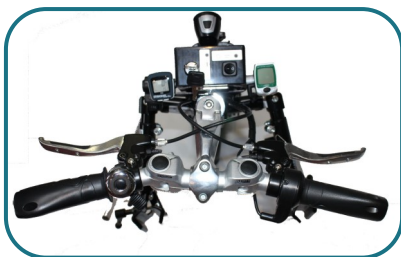
Compteur multifonction + Afficheur de gestion de la batterie
