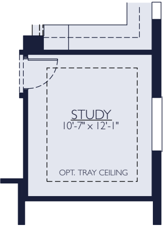
OPT. STUDY IN LIEU OF DINING
