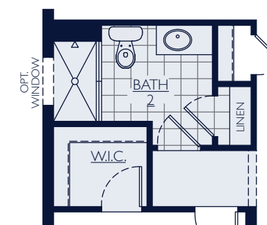
OPT. SHOWER IN LIEU OF TUB BATH 2
