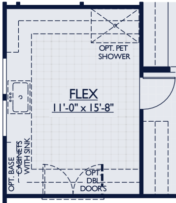
OPT. FLEX IN LIEU OF TANDEM
