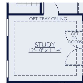
OPT. STUDY IN LIEU OF BEDROOM 2
