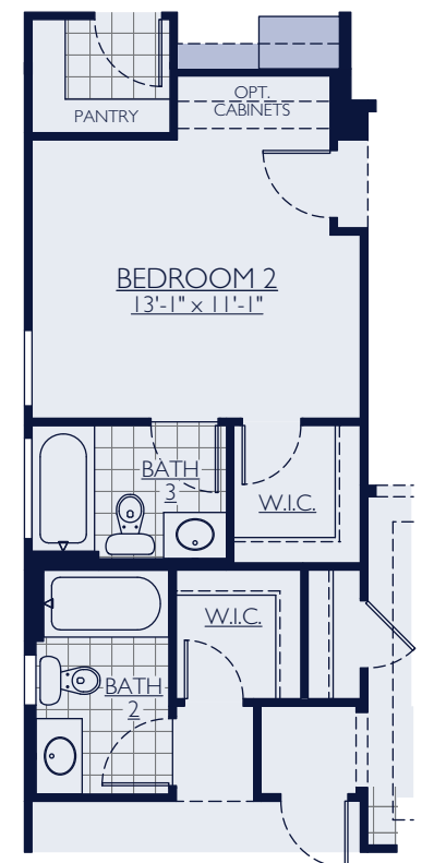
OPT. BEDROOM 2 & 3 SUITES
