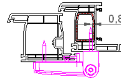
Telaio a Z + m-tec I
