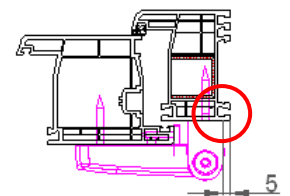
Cerniera Mtec-I / Telaio finestra
