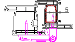
Telaio a Z + m-tec III
