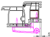
Telaio finestra + m-tec I
