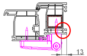
Cerniera Mtec-I / Telaio porta
