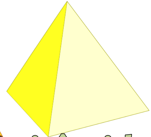
pirâmide quadrangular
