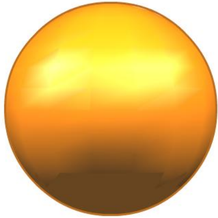
esfera
