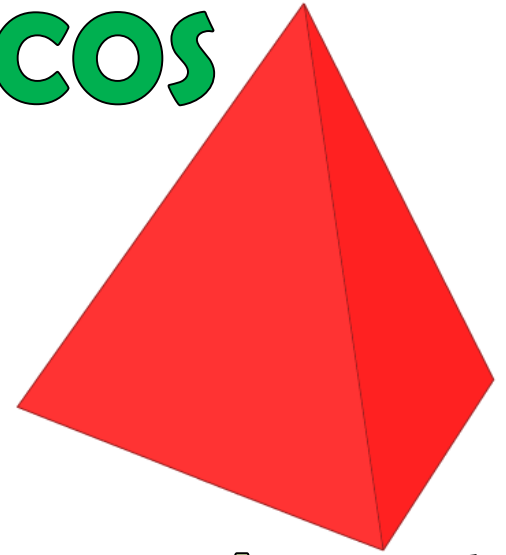
pirâmide triangular
