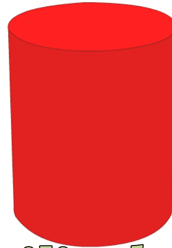
cilindro
