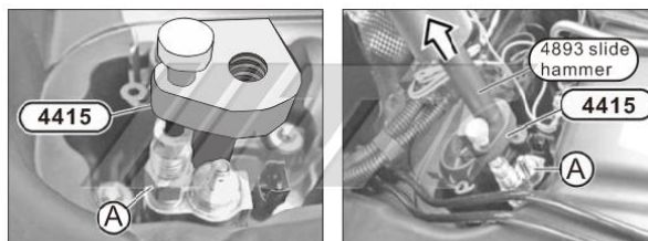
A:injector
