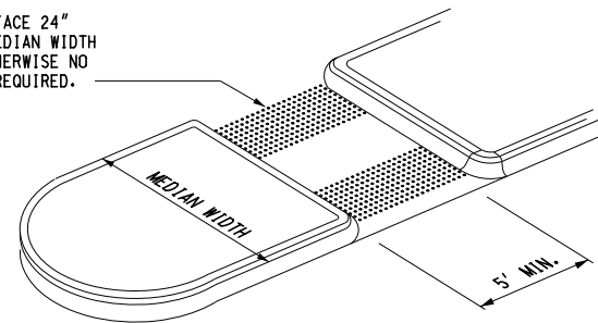
SIDEWALK RAMP TYPE M (MEDIAN ISLAND)
