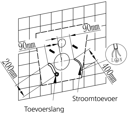
Toevoerslang
