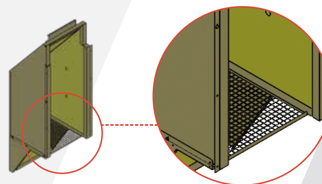
吸込側防音フードに保護網を付けた形状
