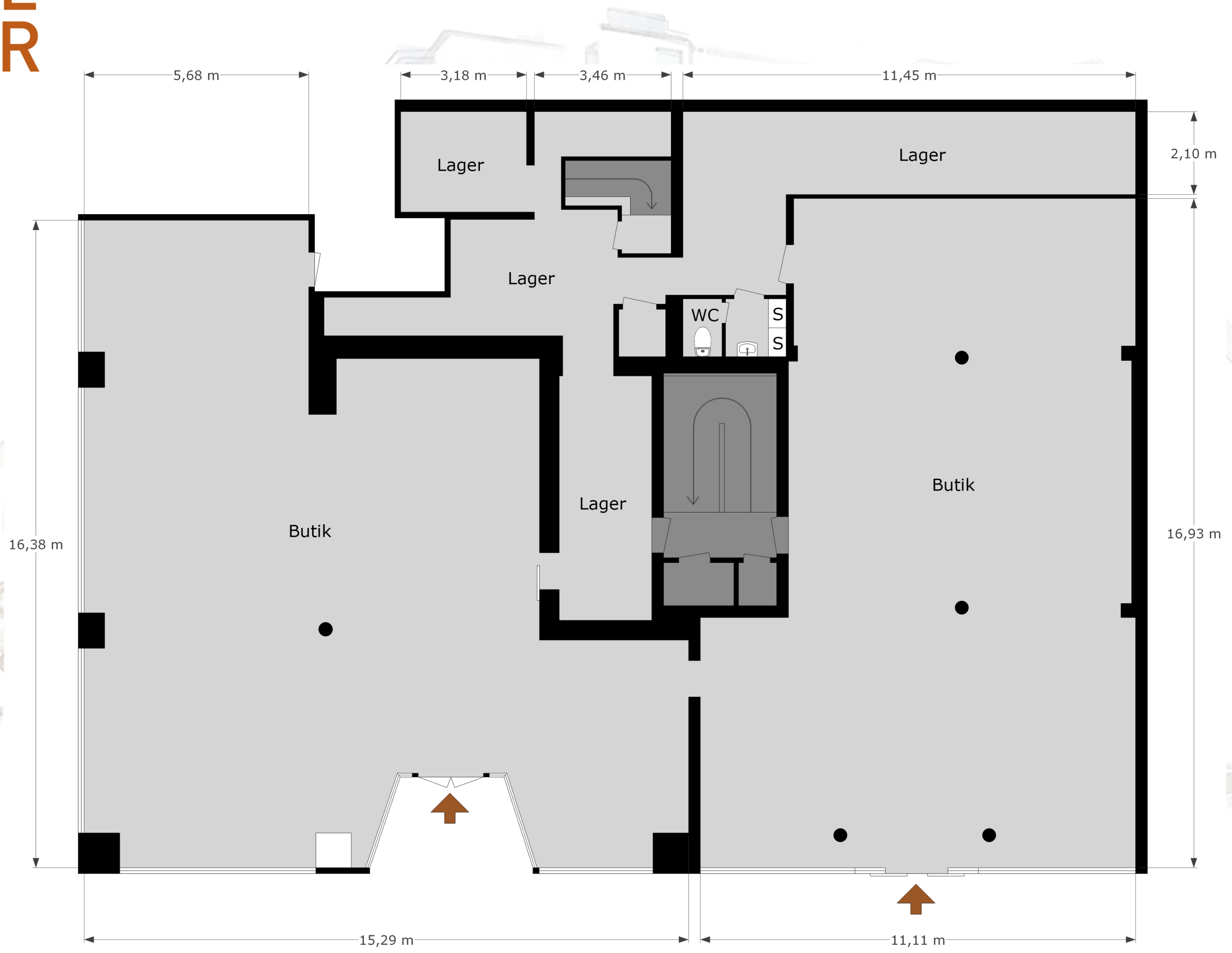
Kungsporsavenyn 17, Entréplan 453,6m 2
